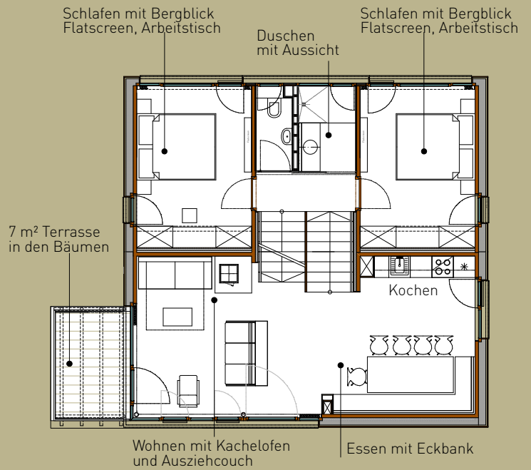
Wohngeschoss 1 ca. 76 m 2
