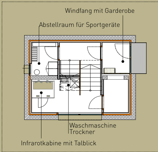
Sockelgeschoss ca. 20 m 2
